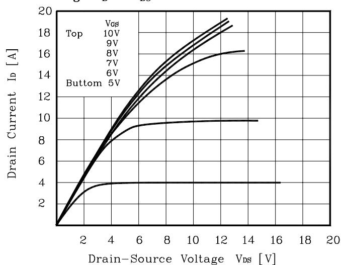
Fig. 1 I_D - V_{DS}
