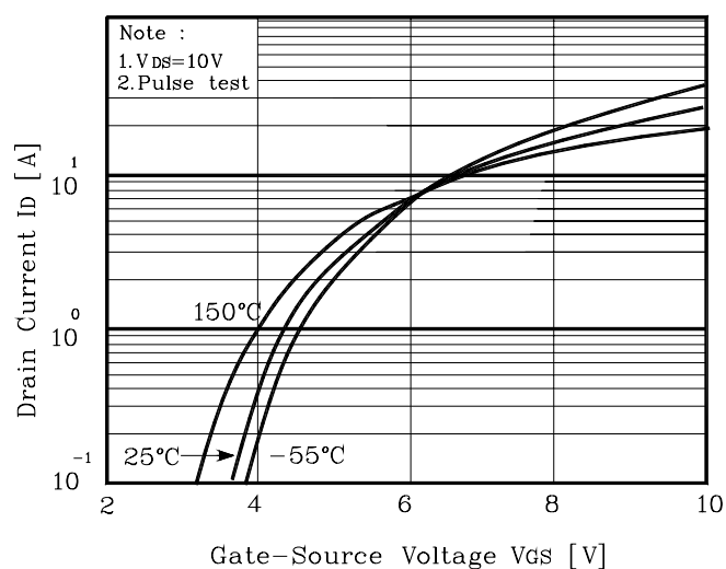
Fig. 2 I_D - V_{GS}
