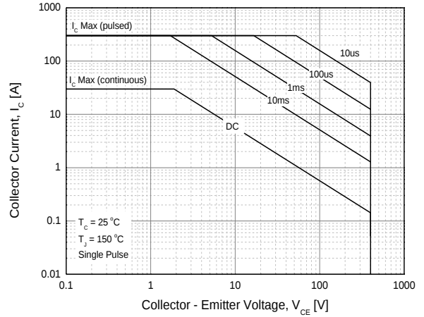
Fig. 14 SOA
