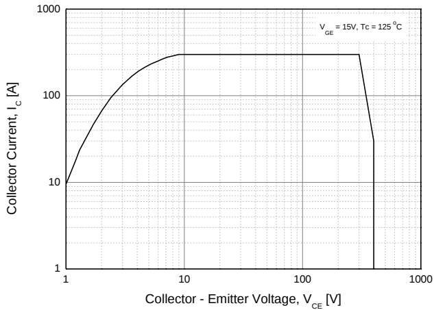
Fig. 15 RBSOA
