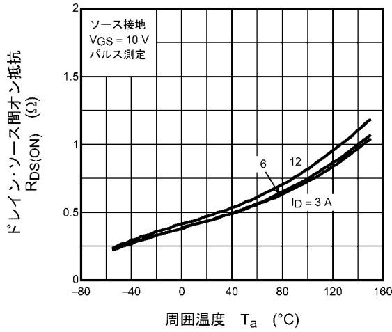
図 8.7 R_{DS(ON)} - T_a
