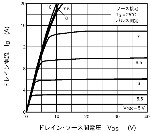
図 8.2 I_D - V_{DS}
