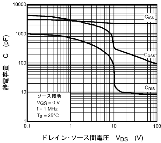
図 8.9 C - V_{DS}
