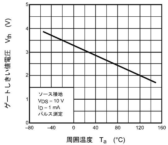
図 8.10 V_{th} - T_a
