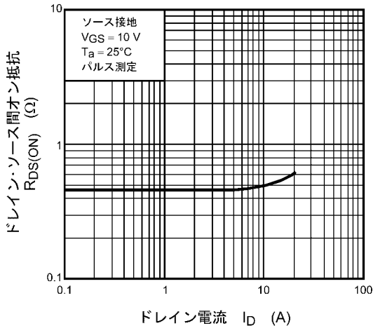
図 8.6 R_{DS(ON)} - I_D
