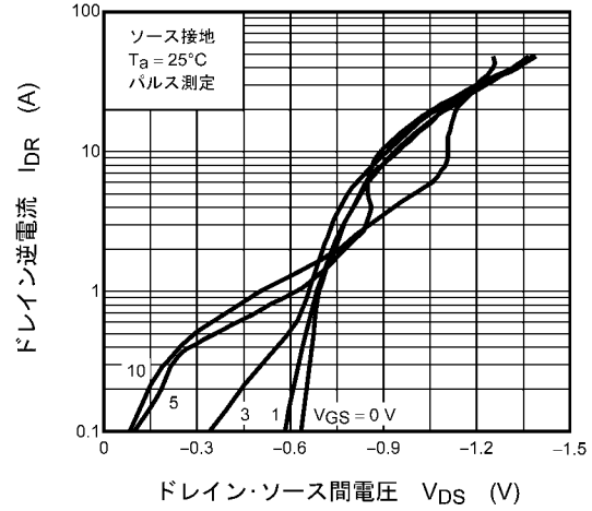
図 8.8 I_{DR} - V_{DS}
