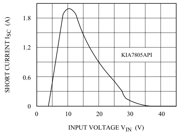
V_{IN} - I_{SC}
