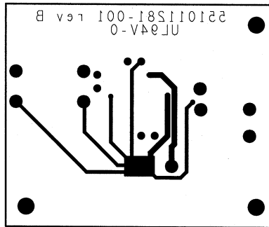
Figure 33. Bottom Layer
