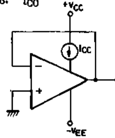
8. I_{CO}
