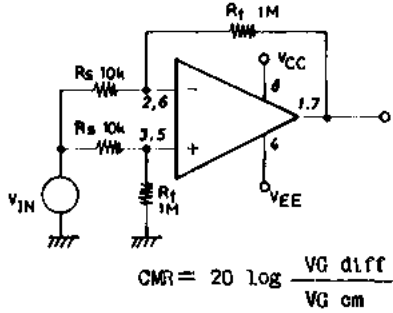
3. V_{ICM}, CMR
