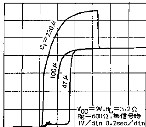
(b) C_1 依存性 C_2 = 100\mu (固定)
