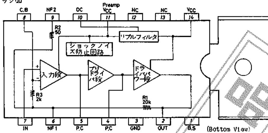
等価回路ブロック図
