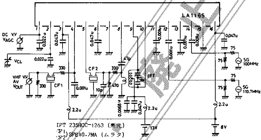
測定回路 3
