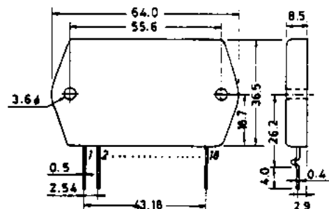
外形図 4050 (unit:mm)
