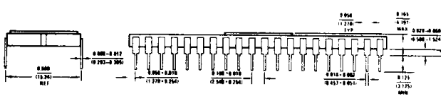
40-Lead Ceramic Dual-in-Line Package (D) Order Number INS8080AD
