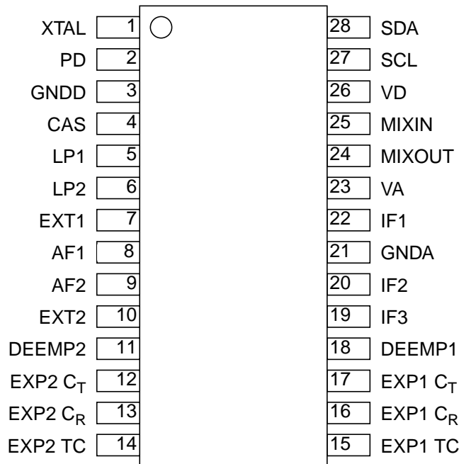
P-DSO 28-1
