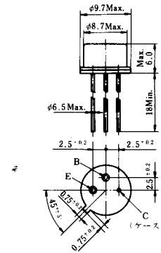
外形寸法 (単位: mm) JEDEC(TO-5), EIAJ(TC-5, TB-5B)
